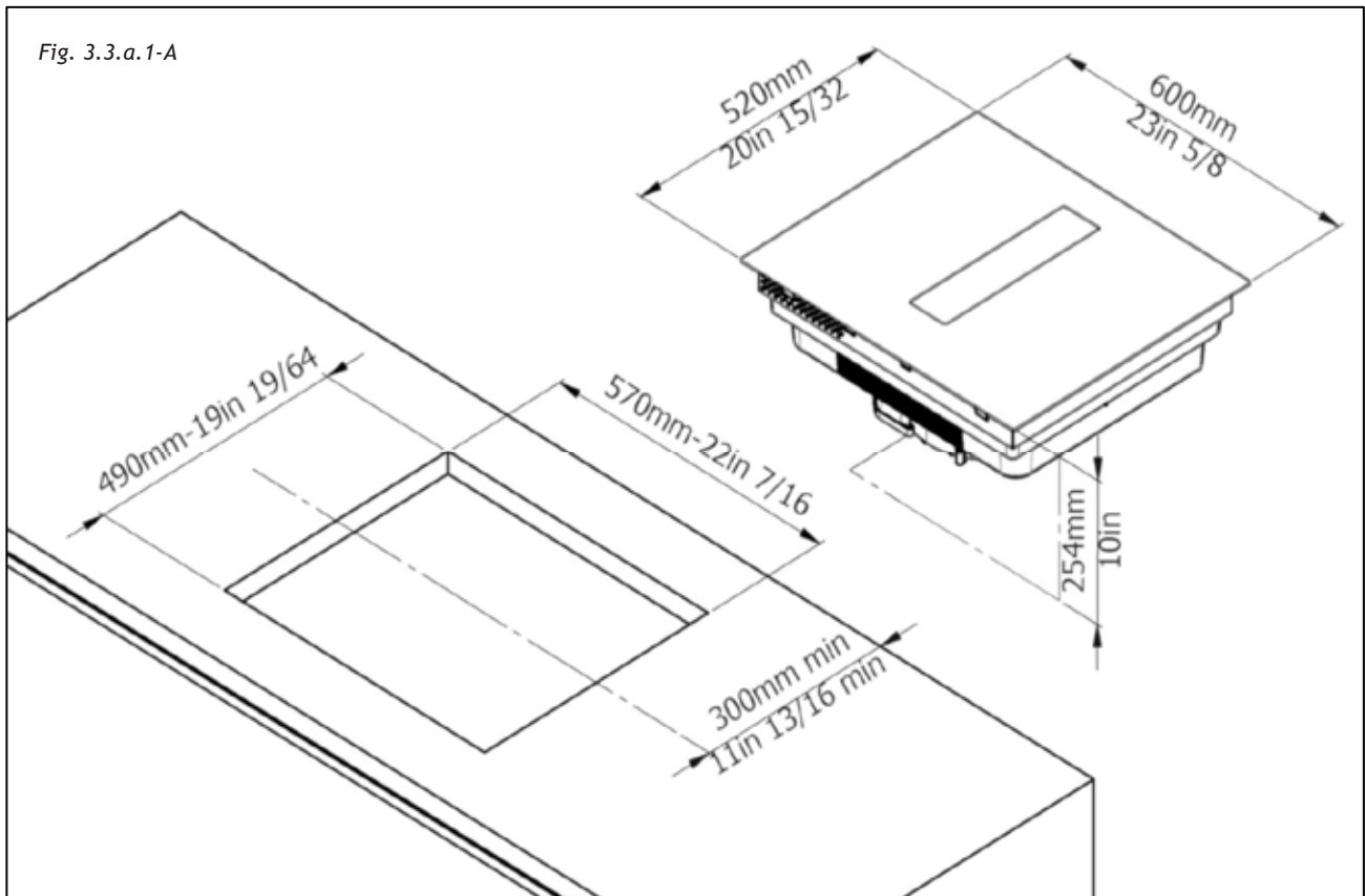
Fig. 3.3.a.1-A -> 60cm-23in 5/8 hob:
